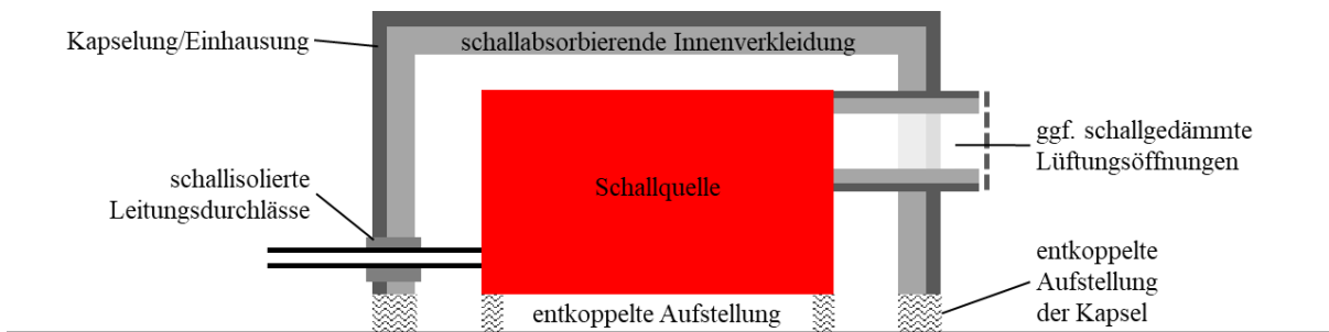
Abbildung 3: schematische Darstellung einer Kapselung
