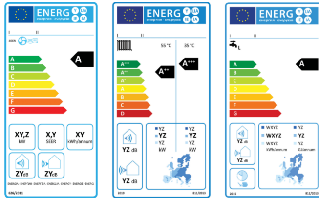
Abbildung 1: Muster des Energielabels für Klimageräte (Verordnung (EU) Nr. 626/2011), für Raumheizungen mit Wärmepumpe (Verordnung (EU) Nr. 811/2013) und für Warmwasserbereiter mit Wärmepumpe (Verordnung (EU) Nr. 812/2013). Der Schalleistungspegel (außen) wird symbolisiert dargestellt ( ) und als „ZY dB“ bzw. „YZ dB“ angegeben.
